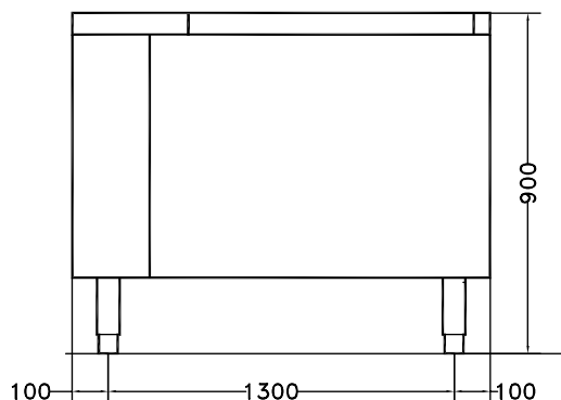
Zij aanzicht
