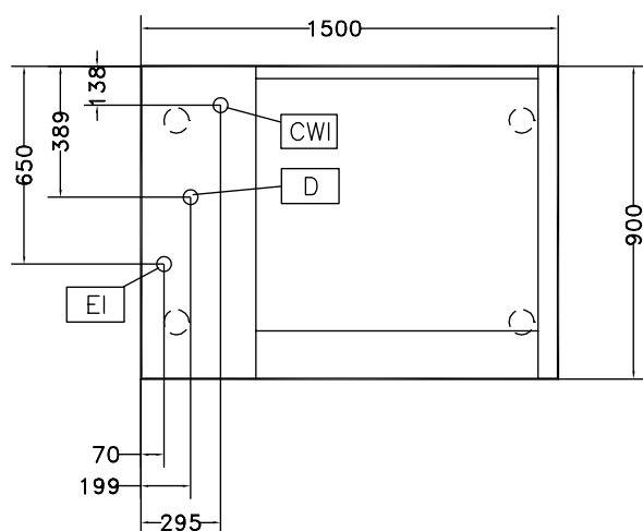
Boven aanzicht
